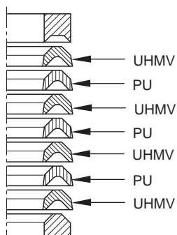
Packing set upper (UHMV + PU) 6004 0266 73
