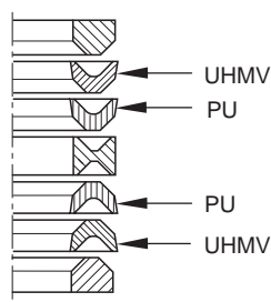
Packing set lower (UHMV + PU) 6004 0266 78
